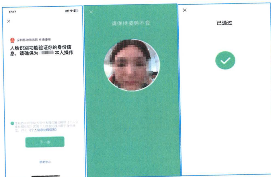
图 1.1-4 人脸识别
