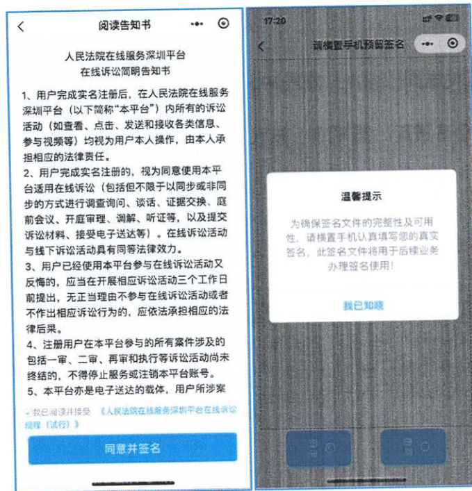
图 1.1-5 在线签名
