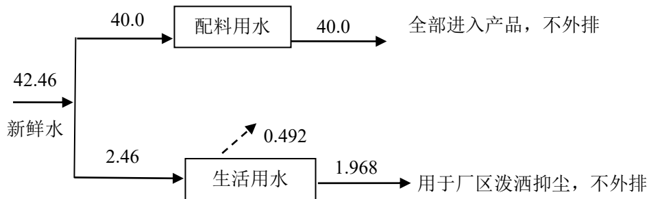
图 2-1 本项目给排水平衡图 单位: m 3 /d
